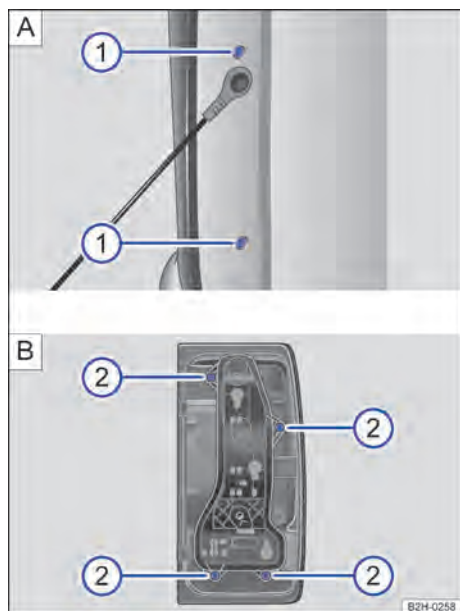
Fig. 198 Suporte da lâmpada.
