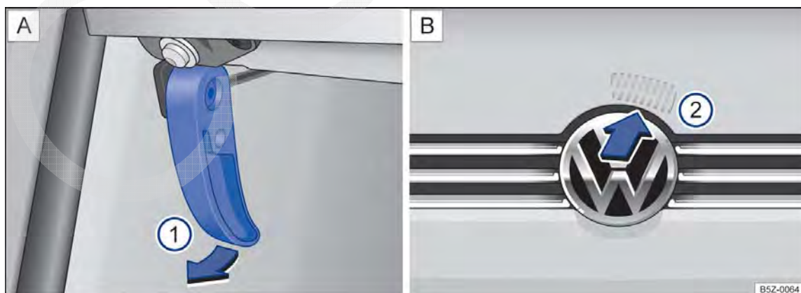
Fig. 127 A: alavanca de destravamento na área para os pés do lado do condutor ①. B: alavanca de destravamento na parte interna da tampa do compartimento do motor ②.
