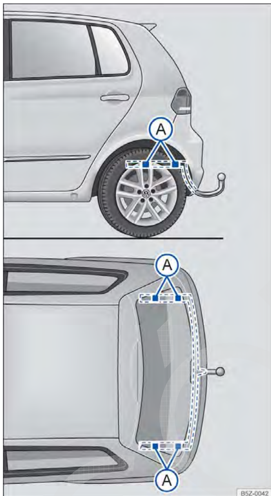
Fig. 82 Pontos de fixação para instalar um dispositivo de reboque posteriormente.
