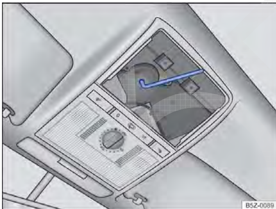
Fig. 159 Parafuso sextavado para fechamento do teto solar.
