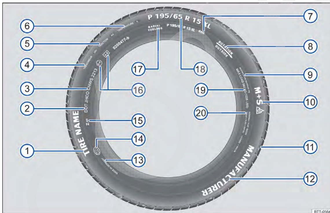
Fig. 144 Inscrição dos pneus internacional (exemplo).
