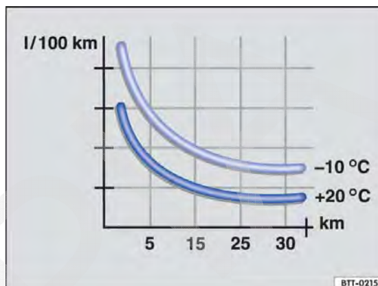
Fig. 113 Consumo de combustível em l/100 km em 2 temperaturas ambiente diferentes.
