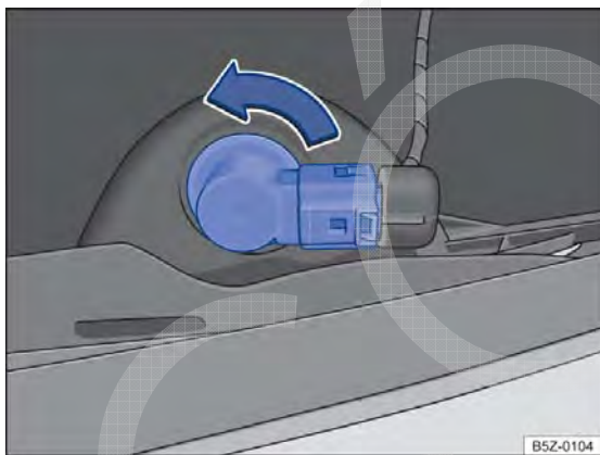
Fig. 182 Atrás do para-choque traseiro: acesso à lâmpada incandescente da lanterna de neblina (somente lado esquerdo).
