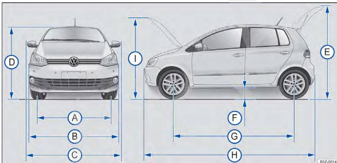
Fig. 19 Dimensões.
