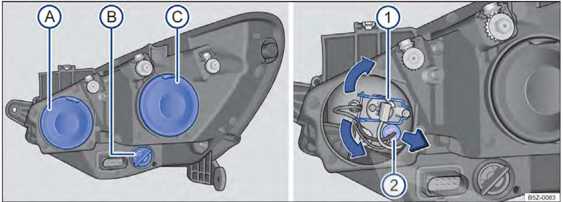
Fig. 174 No compartimento do motor: vista traseira do farol dianteiro direito com cobertura de borracha (esquerda): (A) farol alto e luz de posição, (B) indicadores de direção e (C) farol baixo. Vista traseira do farol dianteiro direito sem cobertura de borracha (direita): (1) farol alto, (2) luz de posição.
