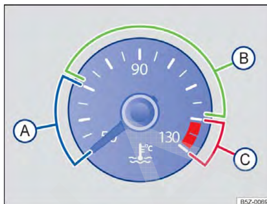
Fig. 131 Indicador de temperatura do líquido de arrefecimento do motor no instrumento combinado: (A) área fria; (B) área normal; (C) área de alerta.
