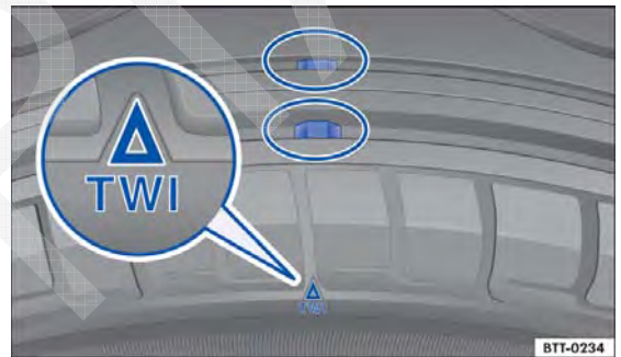
Fig. 142 Perfil do pneu: indicadores de desgaste.
