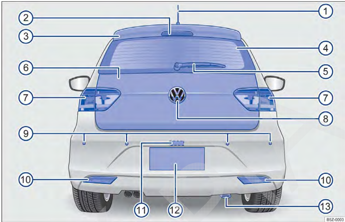
Fig. 3 Vista geral da parte traseira do veículo.
