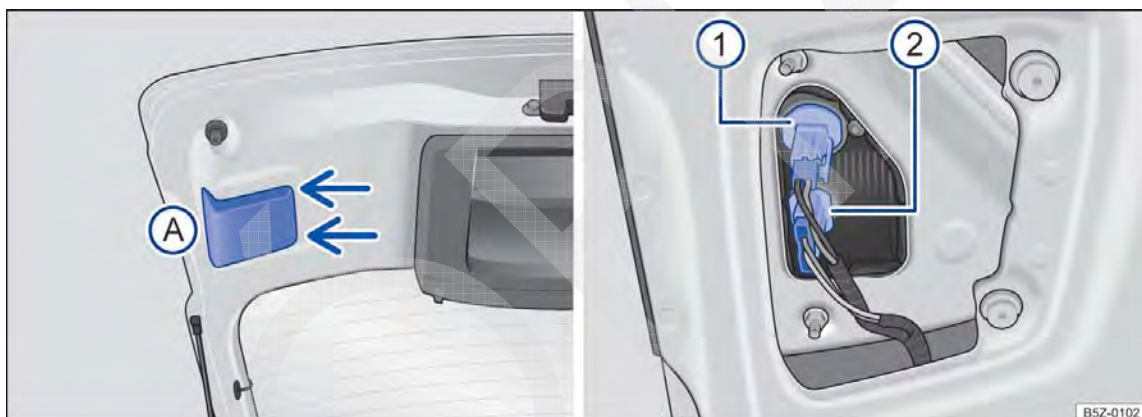
Fig. 181 Lanterna traseira: A desinstalar a cobertura e 1 e 2 desinstalar as lâmpadas.
