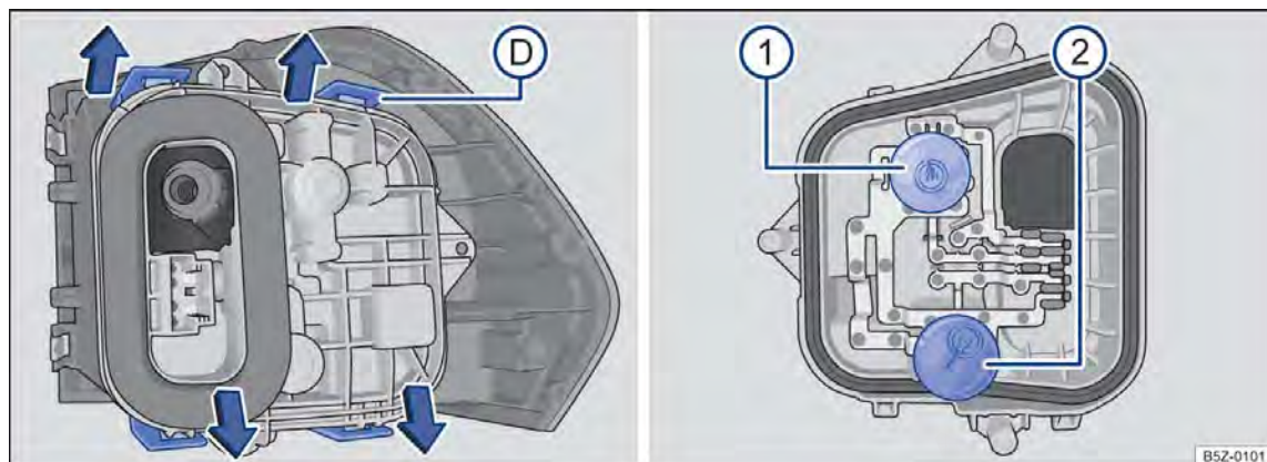
Fig. 180 Lanterna traseira: D desinstalar o suporte das lâmpadas e 1 e 2 desinstalar as lâmpadas incandescentes.
