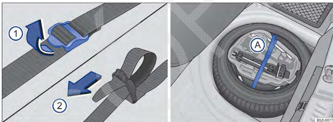
Fig. 161 No compartimento de bagagem: cinta de fixação da caixa de ferramentas e caixa de ferramentas de bordo.
