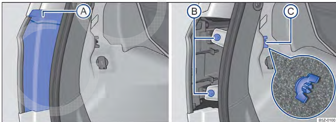
Fig. 179 Lateralmente no compartimento de bagagem: A) desinstalar a cobertura, B) retirar os dois parafusos e C) retirar o parafuso borboleta (lupa).
