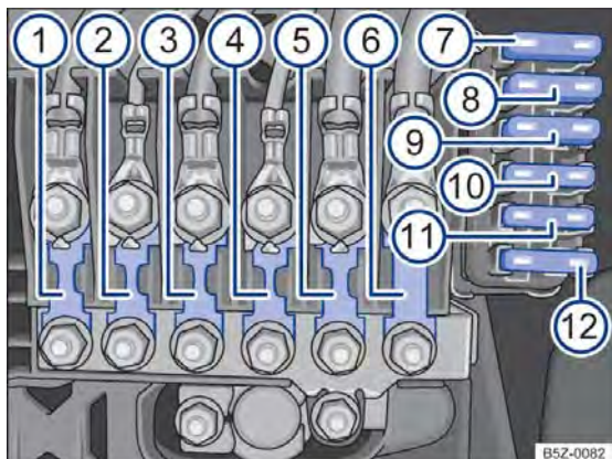
Fig. 173 Caixa de fusíveis.
