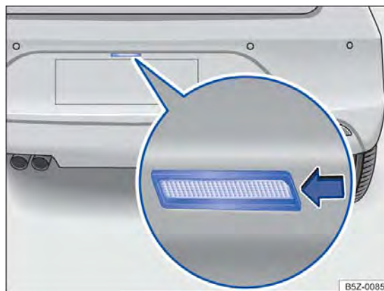
Fig. 183 No para-choque traseiro: remover a lanterna da placa de licença.
