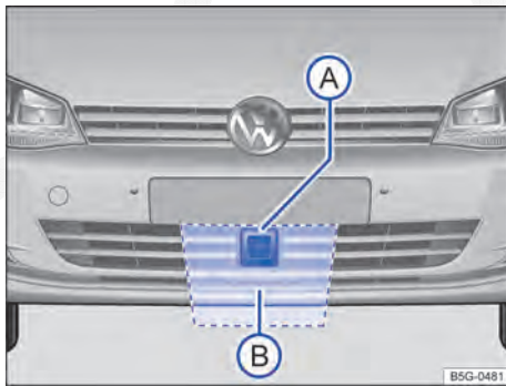
Fig. 162 Na grade do radiador, atrás do logotipo da Volkswagen: sensor do radar e área que deve ser mantida livre em volta do sensor do radar .
