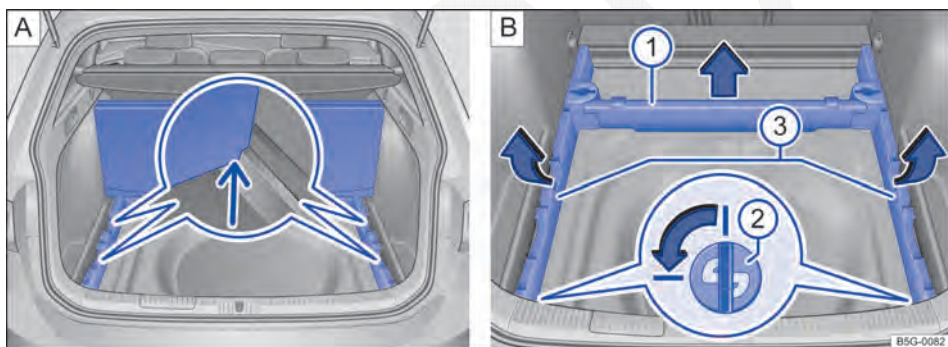
Fig. 103 No compartimento de bagagem: A assoalho do compartimento de bagagem levantado, B remover os suportes do assoalho do compartimento de bagagem.
