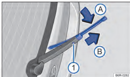
Fig. 188 Substituir a palheta do limpador do vidro traseiro.
