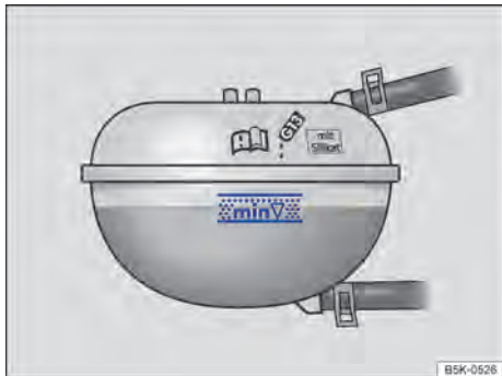
Fig. 177 No compartimento do motor: marcas no reservatório de expansão do líquido de arrefecimento do motor.
