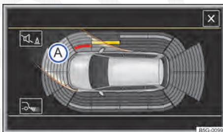
Fig. 140 Exibição do display do Park Pilot: exibição do percurso com ângulo de direção.
