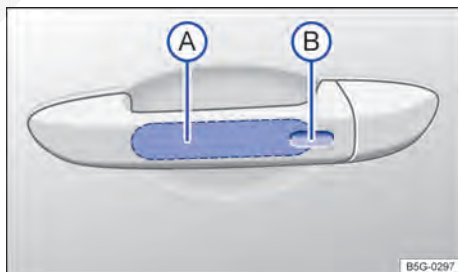
Fig. 27 Sistema de travamento e de partida Keyless Access sem chave: superfície do sensor A para destravamento na parte interna da maçaneta da porta e superfície do sensor B para travamento na parte externa da maçaneta da porta.
