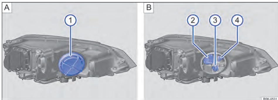
Fig. 221 No compartimento do motor: ① cobertura no farol dianteiro esquerdo, ② farol de conversão, ③ indicadores de direção, ④ luz de posição e farol de rodagem diurna.
