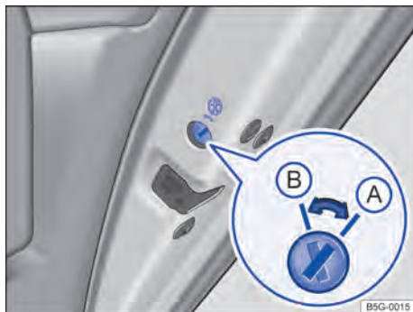
Fig. 31 Na porta traseira direita: trava de segurança para crianças (A) desativada, (B) ativada.
