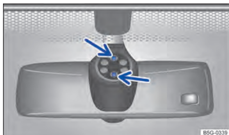
Fig. 87 No para-brisa acima do espelho retrovisor interno: superfícies sensíveis do sensor de chuva e de luz.
