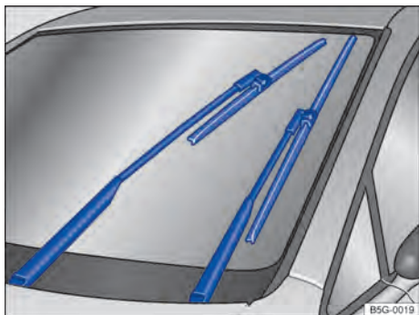
Fig. 85 Limpadores dos vidros na posição de serviço.
