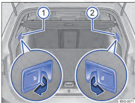
Fig. 52 No compartimento de bagagem: alavanca de destravamento à distância para a parte esquerda ① e a para parte direita ② do encosto do banco traseiro.
