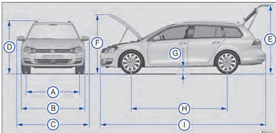
Fig. 235 Dimensões.
