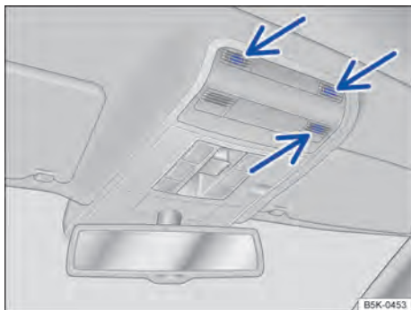
Fig. 29 No console do teto: sensores do monitoramento do interior do veículo (setas).
