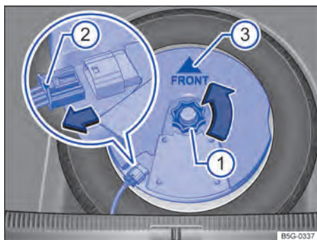
Fig. 214 No compartimento de bagagem: remover o subwoofer (variante 2).
