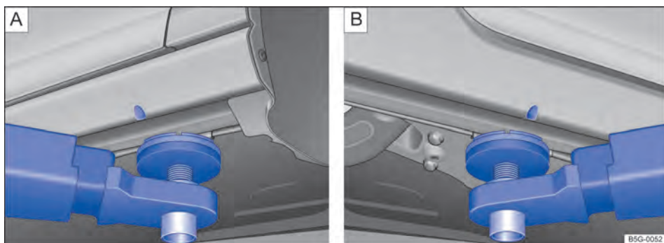
Fig. 189 A Pontos de apoio dianteiros e B ponto de apoio traseiro para suspender com a plataforma elevatória ou o macaco (variante 1).
