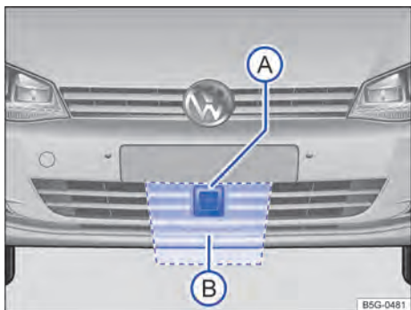
Fig. 156 Na grade do radiador, atrás do logotipo da Volkswagen: sensor do radar (A) e área que deve ser mantida livre em volta do sensor do radar (B).
