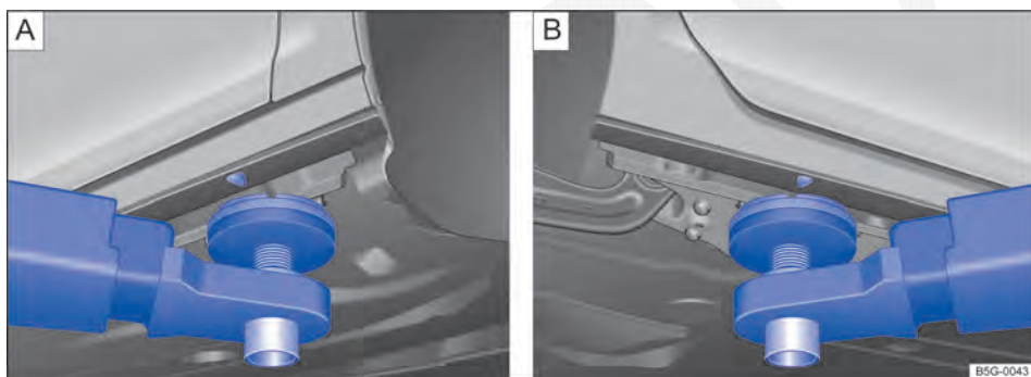
Fig. 190 A Pontos de apoio dianteiros e B ponto de apoio traseiro para suspender com a plataforma elevatória ou o macaco (variante 2).
