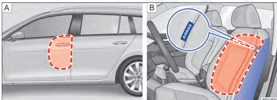
Fig. 68 A No lado esquerdo do veículo: áreas de expansão do airbag lateral. B Lateralmente no banco dianteiro: local de instalação e área de expansão dos airbags laterais.
