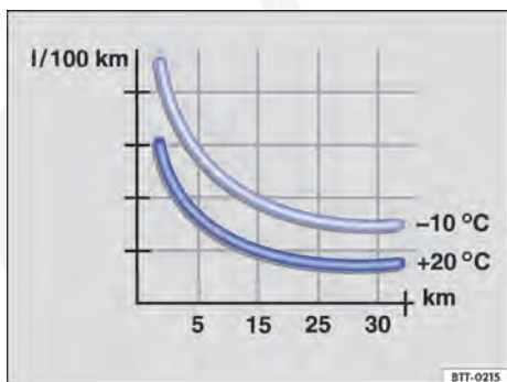
Fig. 133 Consumo de combustível em l/100 km em 2 temperaturas ambiente diferentes.
