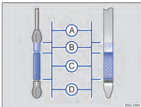
Fig. 174 Vareta de medição do óleo com marcas de nível do óleo do motor (variantes).
