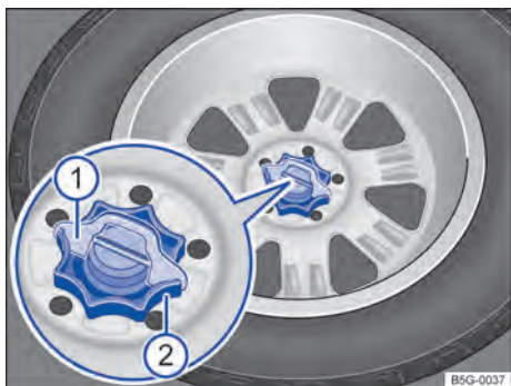
Fig. 185 No compartimento de bagagem: manípulo para fixação da roda sobressalente.
