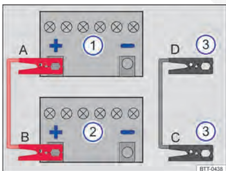
Fig. 228 Esquema para a conexão dos cabos auxiliares de partida no veículo que presta auxílio à partida.
