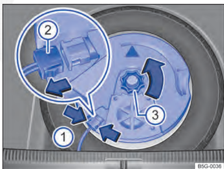
Fig. 213 No compartimento de bagagem: remover o subwoofer (variante 1).
