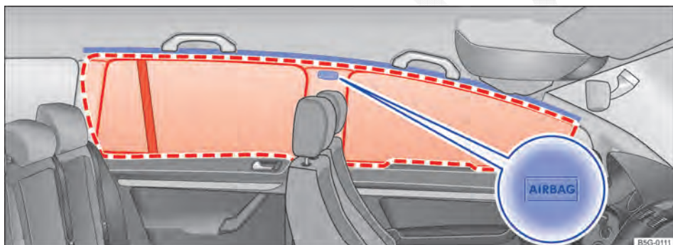
Fig. 69 No lado esquerdo do veículo: local de instalação e área de expansão do airbag para cabeça.
