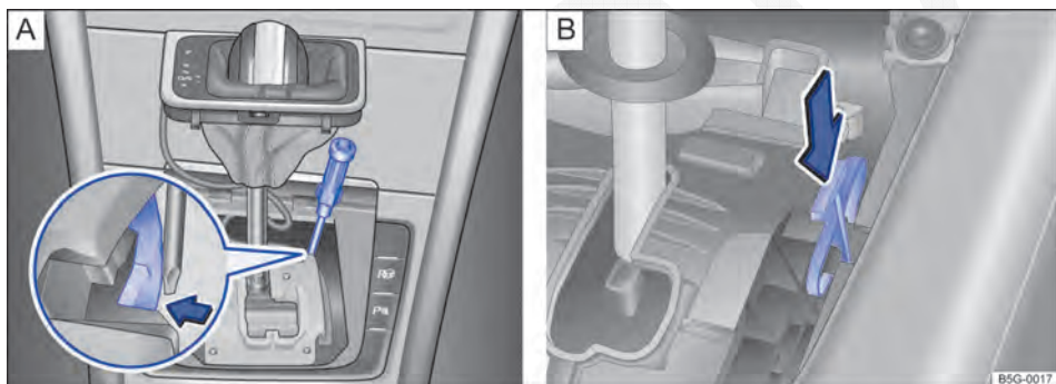
Fig. 199 Embaixo da cobertura do quadro da alavanca seletora: destravar o bloqueio da alavanca seletora emergencialmente (variante A) e (variante B).
