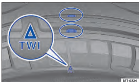
Fig. 184 Perfil do pneu: indicadores de desgaste.
