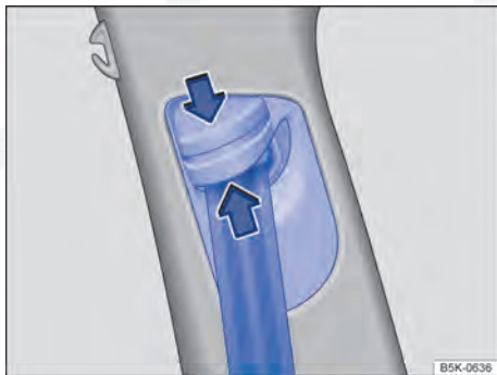
Fig. 63 Ao lado dos bancos dianteiros: regulagem de altura do cinto de segurança.
