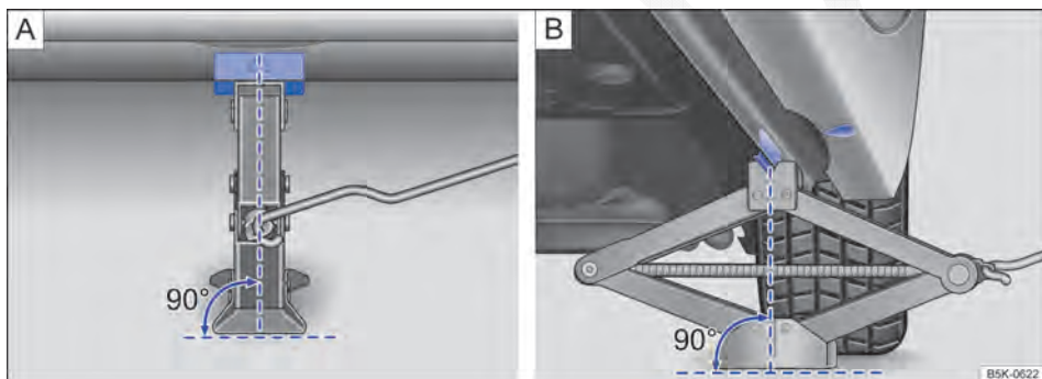
Fig. 212 Macaco posicionado no lado esquerdo traseiro do veículo.
