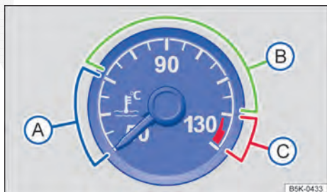
Fig. 176 Indicador da temperatura do líquido de arrefecimento do motor no instrumento combinado: (A) área fria; (B) área normal; (C) área de advertência.
