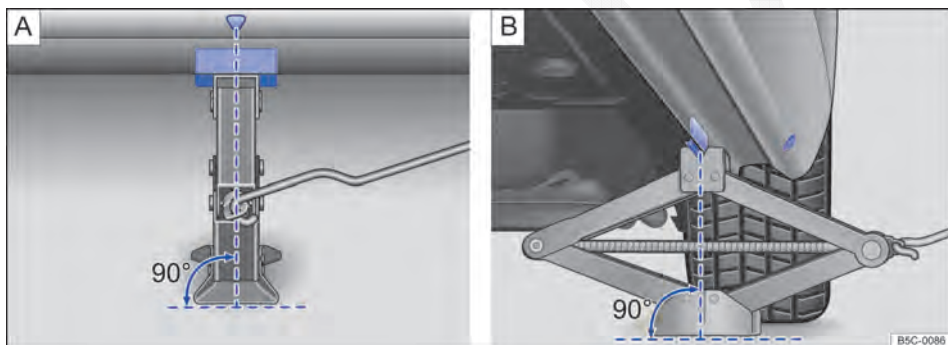
Fig. 210 Macaco posicionado no lado esquerdo traseiro do veículo.
