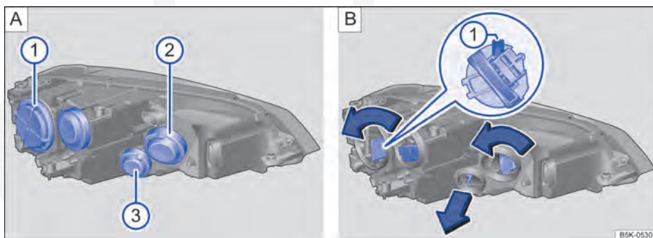
Fig. 220 No compartimento do motor: coberturas do farol dianteiro esquerdo. ① farol baixo, ② farol alto e luz de posição, bem como farol de rodagem diurna, ③ indicador de direção.
