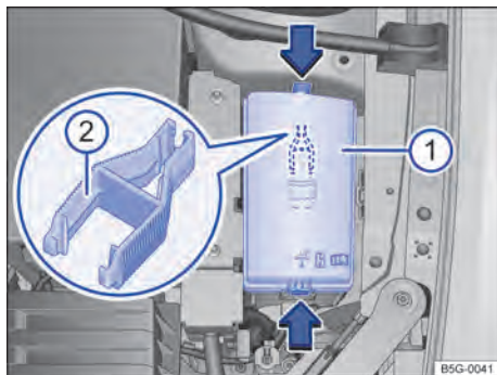
Fig. 217 No compartimento do motor: cobertura (1) da caixa de fusíveis com pinça de plástico (2).
