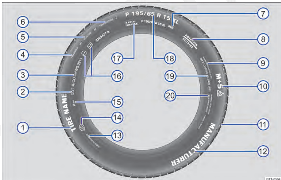
Fig. 186 Inscrição internacional dos pneus.
