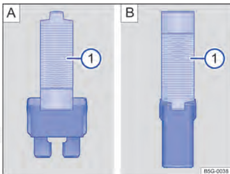
Fig. 219 Retirar ou colocar o fusível com a pinça de plástico: A fusível plano, B fusível de bloqueio.
