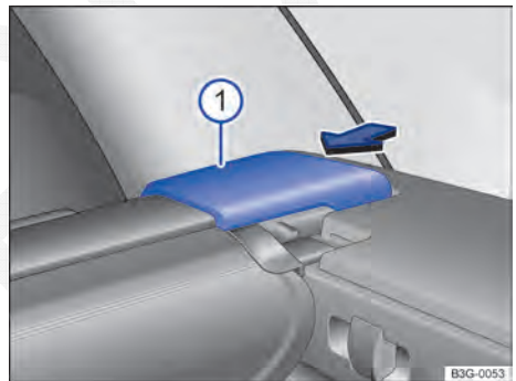
Fig. 93 No compartimento de bagagem: remover a cobertura do compartimento de bagagem.
