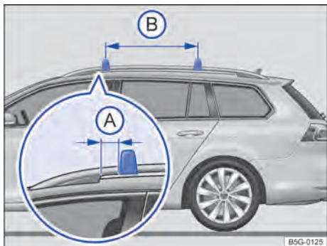
Fig. 104 Longarina do bagageiro do teto: fixação das barras de suporte.
