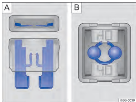
Fig. 218 Fusível queimado: A fusível plano, B fusível de bloqueio.
