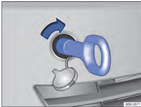
Fig. 220 No para-choque dianteiro à direita: rosquear a argola de reboque.
