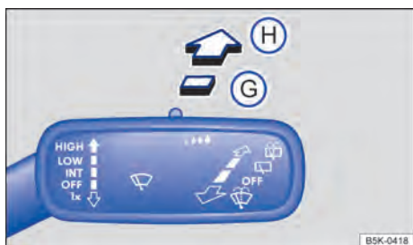
Fig. 74 À direita da coluna de direção: comandar o limpador / lavador do vidro traseiro.
