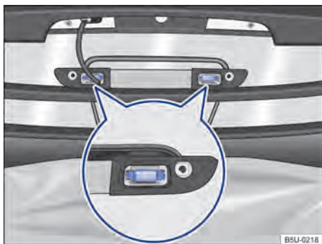
Fig. 190 Lanterna de freio elevada: remover a lâmpada incandescente da iluminação do compartimento de carga.
