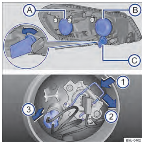
Fig. 180 No compartimento do motor: vista traseira do farol dianteiro com cobertura de borracha (lado esquerdo da ilustração) - A farol baixo, B farol alto e luz de posição, e C indicador de direção. Vista traseira do farol dianteiro sem a cobertura de borracha (lado direito da ilustração): 1 mola de travamento da lâmpada incandescente do farol e 2 luz de posição.
