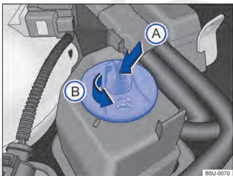
Fig. 116 No compartimento do motor: reservatório do fluido da direção hidráulica.
