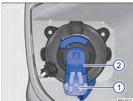
Fig. 191 Trocar a lâmpada incandescente do farol de neblina.
