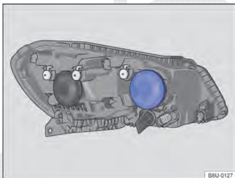
Fig. 186 No compartimento do motor: localização da lâmpada incandescente do farol alto / longo alcance e luz de posição.
