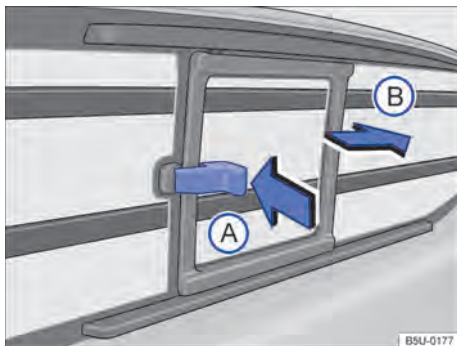
Fig. 39 No compartimento de carga: abertura do vidro corredeço.
