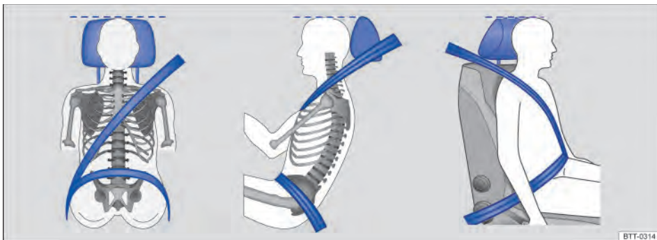
Fig. 56 Posição correta do caderço do cinto de segurança e ajuste correto do apoio para cabeça.
