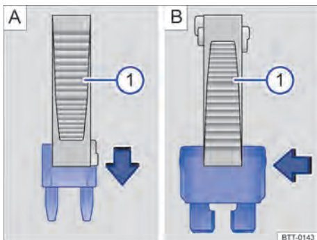
Fig. 175 Remover ou instalar um fusível com a garra da pinça de plástico ①.
