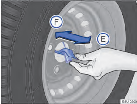
Fig. 167 Na roda de emergência: remover o cabo do aro da roda de emergência.
