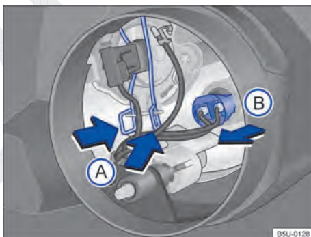
Fig. 187 Acesso à lâmpada incandescente do farol alto / longo alcance e luz de posição.
