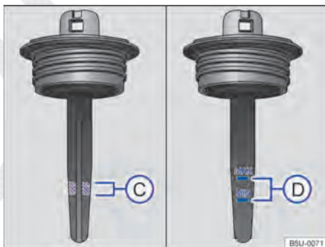
Fig. 117 Marcações para controle do nível do fluido da direção hidráulica.
