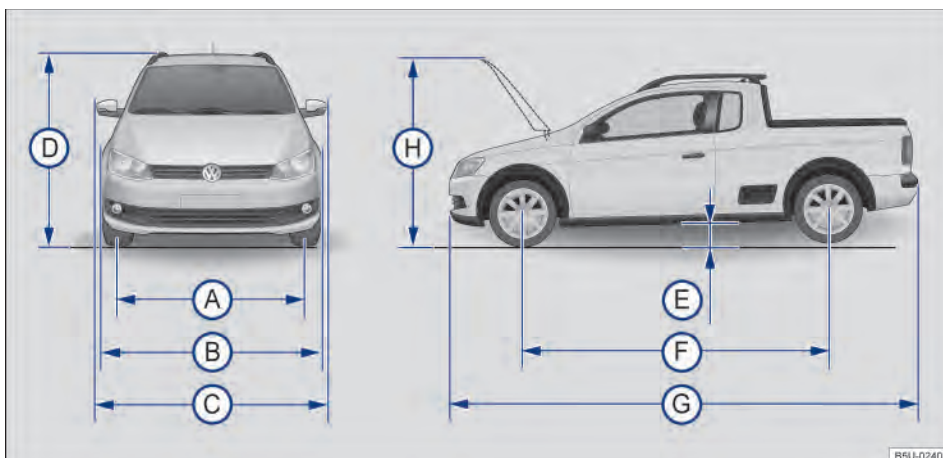
Fig. 20 Dimensões.
