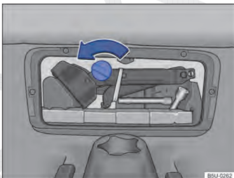
Fig. 161 Manípulo de fixação da caixa de ferramentas de bordo.
