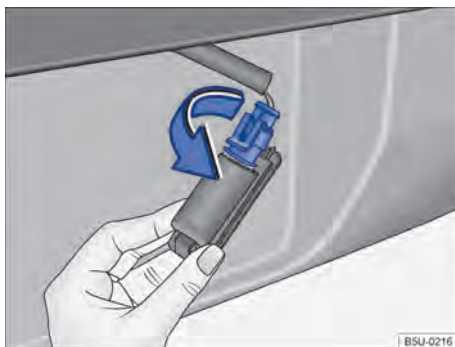
Fig. 197 Lanterna da placa de licença: remover o soquete da lâmpada.
