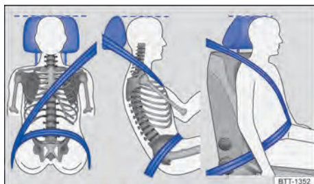
Fig. 62 Posição correta do caderço do cinto de segurança e ajuste correto do apoio para cabeça.
