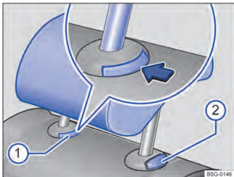
Fig. 45 Assento traseiro central: remover o apoio para cabeça.
