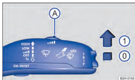
Fig. 85 Alavanca dos limpadores do para-brisa: regular a sensibilidade do sensor de chuva e de luz A .
