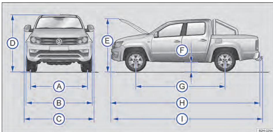
Fig. 213 Dimensões.
