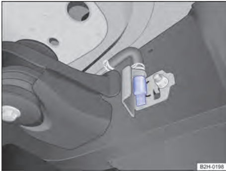
Fig. 137 Parte inferior do veículo na longarina: bujão de drenagem.
