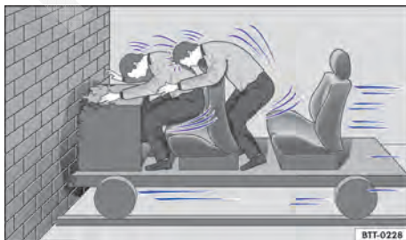
Fig. 5 Um veículo com os ocupantes do veículo sem cintos de segurança colide com o muro.
