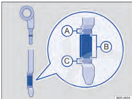
Fig. 159 Varetas de medição do óleo com marcas de nível do óleo do motor.
