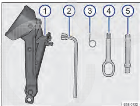
Fig. 131 Representação esquemática: componentes das ferramentas de bordo.
