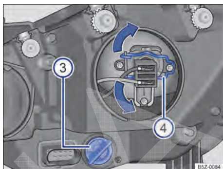
Fig. 136 No compartimento do motor: vista traseira do farol dianteiro direito sem cobertura de borracha: 3 indicadores de direção e 4 farol baixo.
