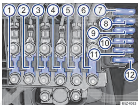
Fig. 148 Caixa de fusíveis.
