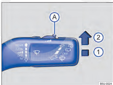
Fig. 75 Ao lado do volante: alavanca dos limpadores dos vidros: regular a sensibilidade do sensor de chuva A .
