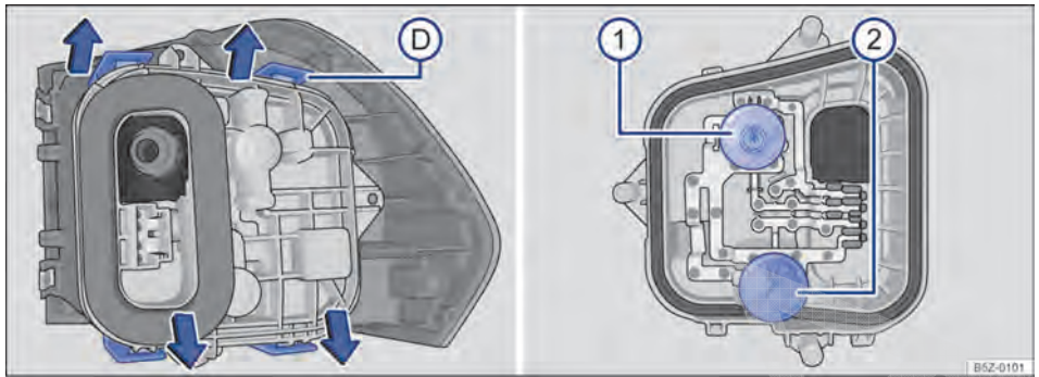
Fig. 140 Lanterna traseira: D desinstalar o suporte das lâmpadas e 1 e 2 desinstalar as lâmpadas incandescentes.
