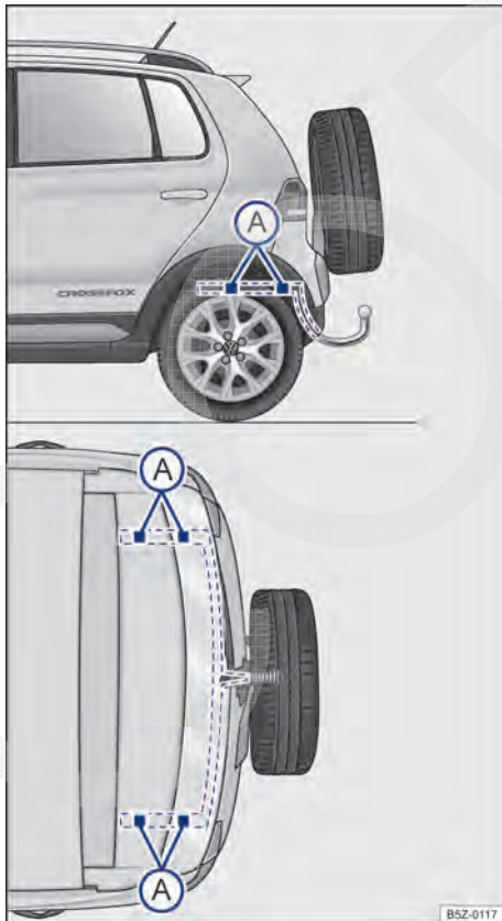
Fig. 127 Pontos de fixação para instalar um dispositivo de reboque posteriormente.
