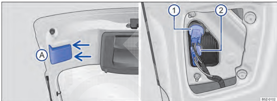
Fig. 141 Lanterna traseira: (A) desinstalar a cobertura e (1) e (2) desinstalar as lâmpadas.
