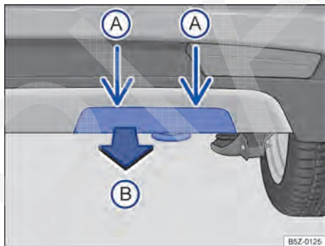
Fig. 155 No para-choque traseiro à direita: argola de reboque traseira - para-choque com cobertura removível.
