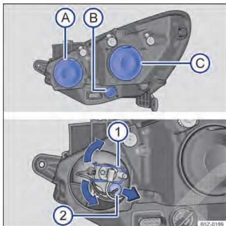
Fig. 135 No compartimento do motor: vista traseira do farol dianteiro direito com cobertura de borracha (esquerda): A farol alto e luz de posição, B indicadores de direção e C farol baixo. Vista traseira do farol dianteiro direito sem cobertura de borracha (direita): 1 farol alto, 2 luz de posição.
