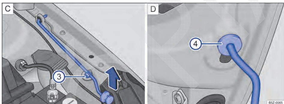
Fig. 157 C: haste de sustentação da tampa do compartimento do motor ③. D: tampa do motor protegida com a haste de sustentação da tampa ④.
