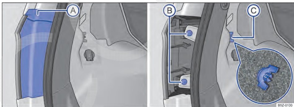
Fig. 139 Lateralmente no compartimento de bagagem: A desinstalar a cobertura, B retirar os dois parafusos e C retirar o parafuso borboleta (lupa).
