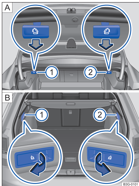
Fig. 93 No compartimento de bagagem: alavanca de destravamento à distância para a parte esquerda ① e parte direita ② do encosto do banco no Passat A e no Passat Variant B .
