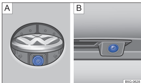
Fig. 270 Na traseira do veículo: câmera de marcha a ré [A] no logo Volkswagen ou [B] na lanterna da placa de licença (representação esquemática).
