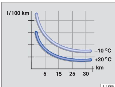
Fig. 126 Consumo de combustível em l/100 km em duas temperaturas ambiente diferentes.
