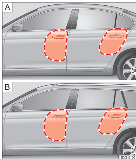
Fig. 47 No lado esquerdo do veículo: áreas de expansão do airbag lateral.
