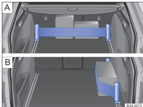
Fig. 197 No compartimento de bagagem: [A] cinta de fixação fixada sobre dois trilhos. [B] Cinta de fixação fixada sobre um trilho (representação esquemática).
