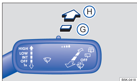
Fig. 109 À direita da coluna de direção: comandar os limpadores do vidro traseiro (Passat Variant).
