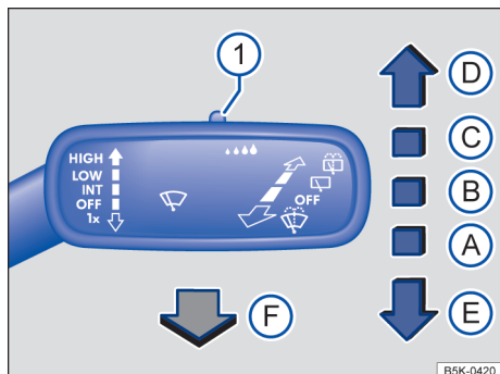
Fig. 108 À direita da coluna de direção: comandar os limpadores do para-brisa.
