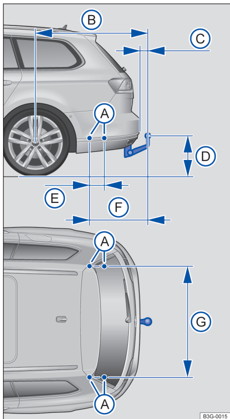
Fig. 208 Dimensões e pontos de fixação para instalação posterior de um dispositivo de reboque (Passat Variant).
