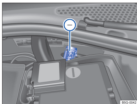
Fig. 230 No compartimento do motor: ponto de auxílio à partida (ponto de aterramento).
