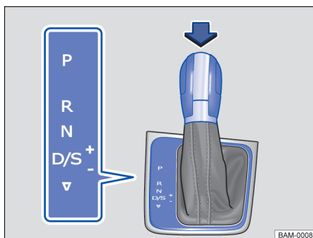
Fig. 132 Veículos com direção à esquerda: alavanca seletora da transmissão automática DSG® com botão bloqueador (seta). Em veículos com direção à direita, a disposição dos elementos é espelhada.
