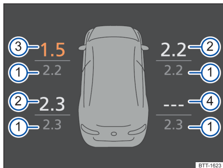
Fig. 249 Representação esquemática do indicador do display no instrumento combinado: pressões dos pneus atuais.
