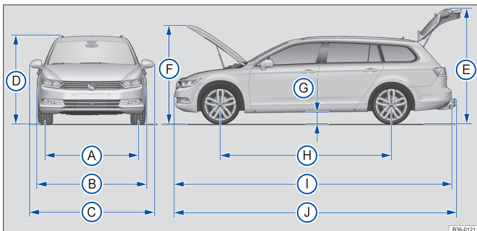
Fig. 274 Dimensões (Passat Variant e Passat Alltrack).
