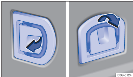
Fig. 192 No compartimento de bagagem: olhal de amarração rebatível.
