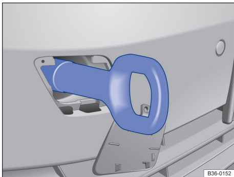
◀ Fig. 237 No para-choque dianteiro à direita: argola de reboque rosqueada.
