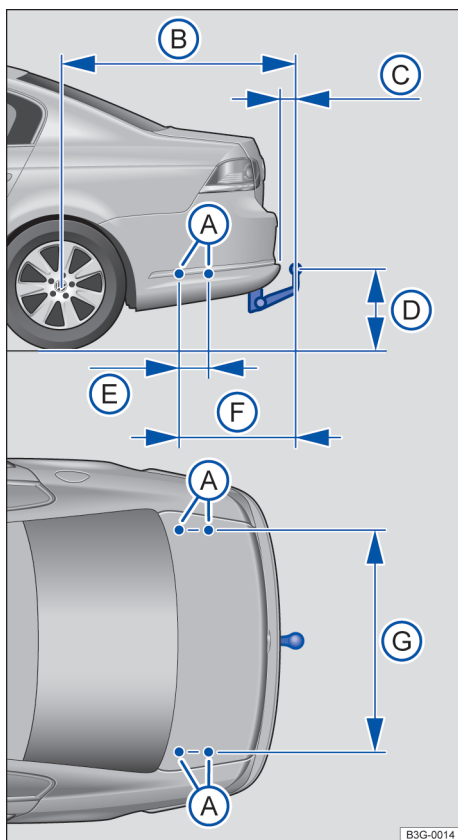
Fig. 207 Dimensões e pontos de fixação para instalação posterior de um dispositivo de reboque (Passat).
