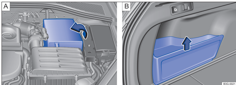
Fig. 247 A No compartimento do motor, B no compartimento de bagagem: A rebater para fora a guarnição da bateria do veículo 12 V, B remover a cobertura da bateria do veículo 12 V.
