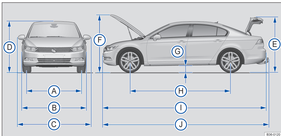
Fig. 273 Dimensões (Passat).
