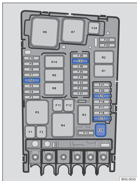
Fig. 227 No compartimento do motor: locais de conexão para fusíveis
