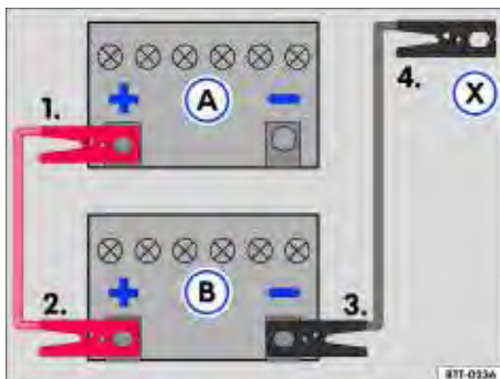
Fig. 192 Esquema para a conexão dos cabos auxiliares de partida: bateria do veículo descarregada e bateria do veículo fornecedora de corrente .
