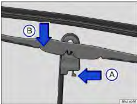
Fig. 133 Substituir as palhetas dos limpadores do para-brisa.
