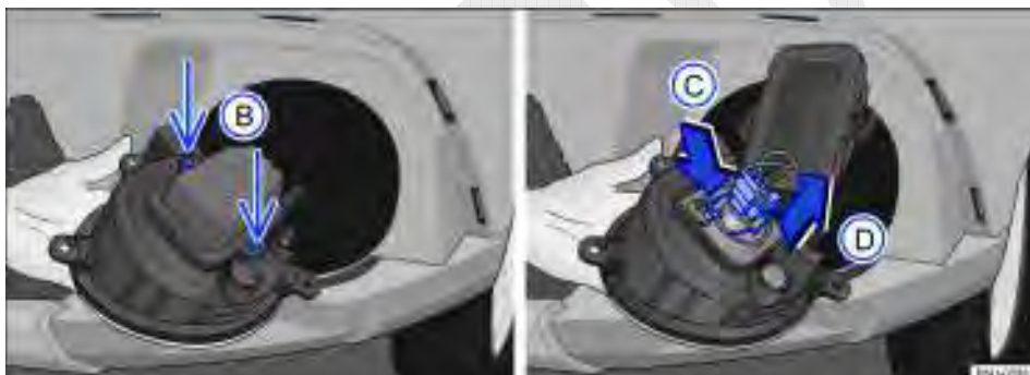
Fig. 185 Remover a cobertura para acesso da lâmpada e acesso a lâmpada do farol de neblina.
