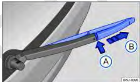
Fig. 134 Substituir a palheta do limpador do vidro traseiro.
