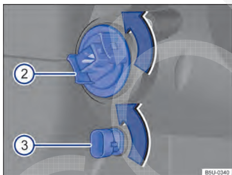
Fig. 200 No compartimento do motor: vista traseira do farol dianteiro (2) indicadores de direção e (3) luz de posição.
