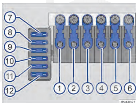
Fig. 198 Caixa de fusíveis.
