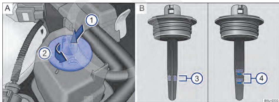
Fig. 130 No compartimento do motor (variante 1): A Reservatório do fluido da direção hidráulica. B Marcações para controle do nível do fluido da direção hidráulica.
