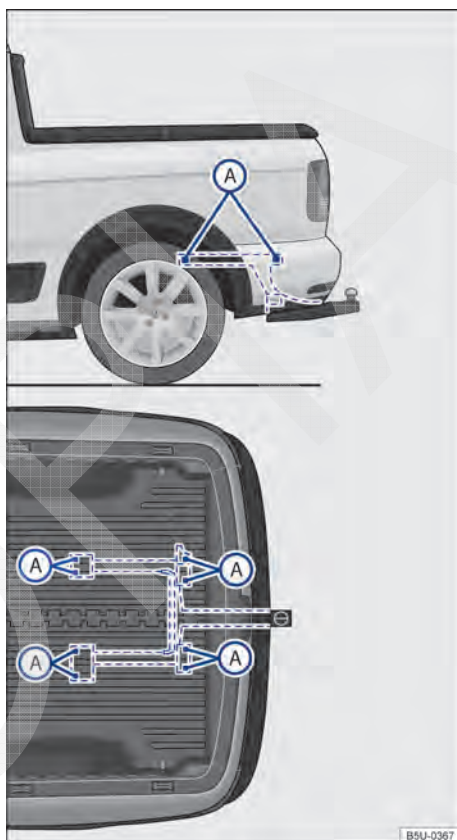
Fig. 96 Pontos de fixação para instalar um dispositivo de reboque posteriormente.
