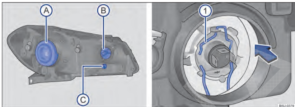
Fig. 199 No compartimento do motor: vista traseira do farol dianteiro com cobertura de borracha (lado esquerdo da ilustração) - (A) farol baixo / alto, (B) indicadores de direção e (C) luz de posição. Vista traseira do farol dianteiro sem a cobertura de borracha (lado direito da ilustração): (1) mola de travamento da lâmpada incandescente do farol baixo / alto.
