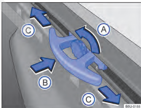
Fig. 91 No compartimento de carga: suporte deslizante para veículos com capota marítima.
