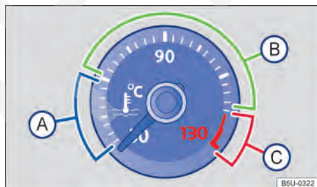
Fig. 154 Indicador de temperatura do líquido de arrefecimento do motor no instrumento combinado (variante 2): (A) área fria; (B) área normal; (C) área de alerta.
