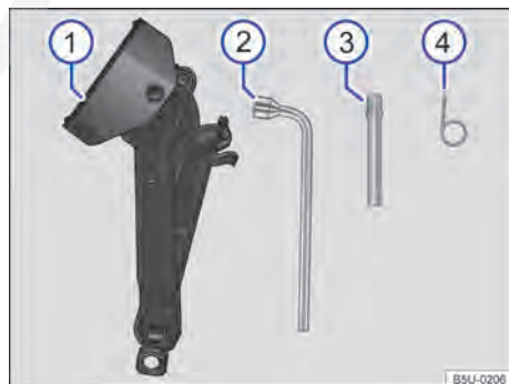
Fig. 192 Componentes das ferramentas de bordo.
