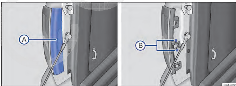
Fig. 206 No compartimento de carga: A desinstalar cobertura, B retirar os parafusos de fixação. ▶
