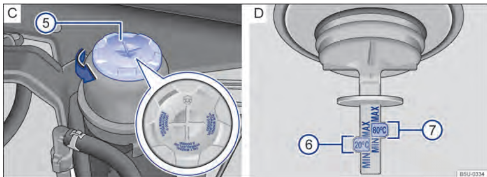
Fig. 131 No compartimento do motor (variante 2): C Reservatório do fluido da direção hidráulica. D Marcações para controle do nível do fluido da direção hidráulica.
