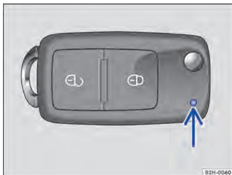
Fig. 25 Luz de controle da chave do veículo com comando remoto.
