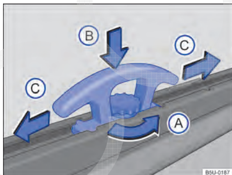
Fig. 90 No compartimento de carga: suporte deslizante para veículos sem capota marítima.
