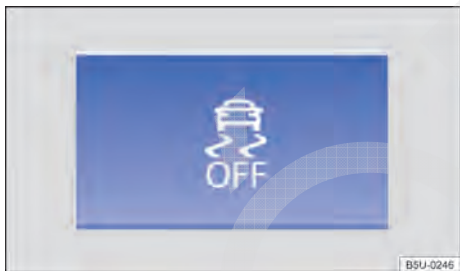
Fig. 127 No console central: botão para desligar e ligar ASR manualmente.
