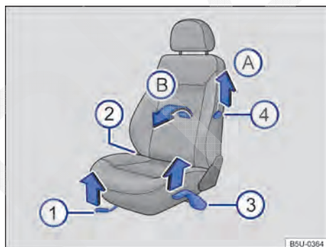
Fig. 44 Comandos do banco esquerdo.
