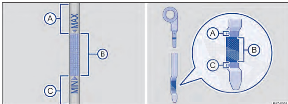
Fig. 151 Vareta de medição do óleo com marcas de nível do óleo do motor.
