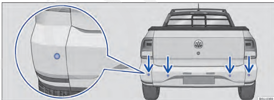
Fig. 135 Sensores de ultrassom do controle de distância de estacionamento no para-choque traseiro.
