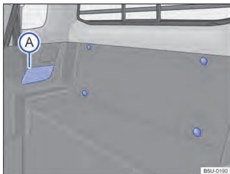
Fig. 93 No compartimento interno de bagagem: (A) grade de exaustão e suportes de amarração da bagagem.
