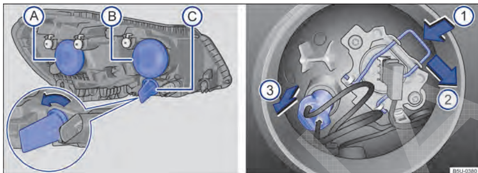
Fig. 201 No compartimento do motor: vista traseira do farol dianteiro com cobertura de borracha (lado esquerdo da ilustração) - (A) farol baixo, (B) farol alto e luz de posição, e (C) indicador de direção. Vista traseira do farol dianteiro sem a cobertura de borracha (lado direito da ilustração): (1) mola de travamento da lâmpada incandescente do farol e (2) luz de posição.
