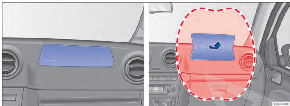
Fig. 67 Local de instalação e área de expansão do airbag frontal do passageiro.
