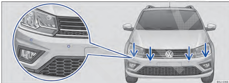
Fig. 134 Sensores de ultrassom do controle de distância de estacionamento no para-choque dianteiro.
