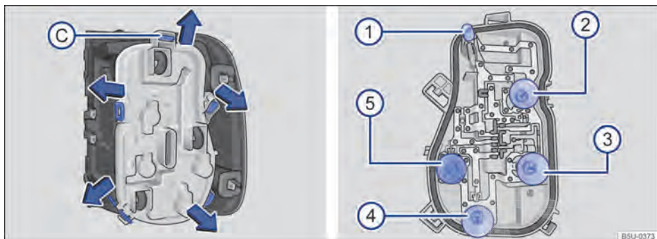
Fig. 207 Lanterna traseira: C desinstalar o suporte das lâmpadas e 1 , 2 , 3 , 4 e 5 desinstalar as lâmpadas.
