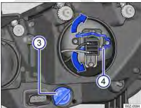
Fig. 175 No compartimento do motor: vista traseira do farol dianteiro direito sem cobertura de borracha: ③ indicadores de direção e ④ farol baixo.
