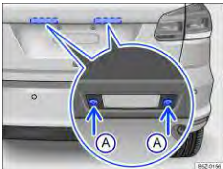
Fig. 183 Na tampa do compartimento de bagagem: remover a lanterna da placa de licença.
