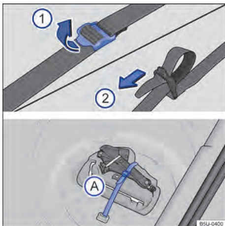
Fig. 123 No compartimento de bagagem: cinta de fixação da caixa de ferramentas e caixa de ferramentas de bordo.
