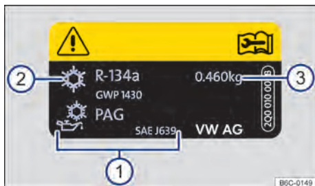
Fig. 174 Informações do ar-condicionado - motor 1.0L TSI e motor 1.6L.
