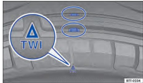
Fig. 197 Perfil do pneu: indicadores de desgaste.
