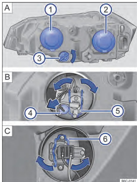
Fig. 166 No compartimento do motor: ① farol alto e luz de posição, ② farol baixo e ③ indicador de direção.
