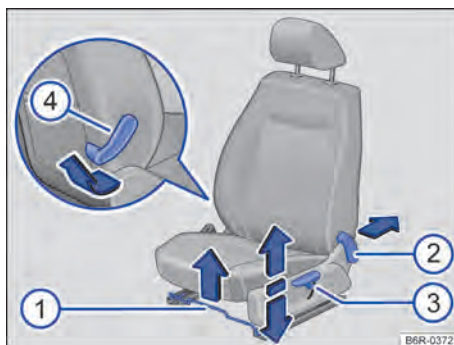
Fig. 64 No banco dianteiro: comandos.
